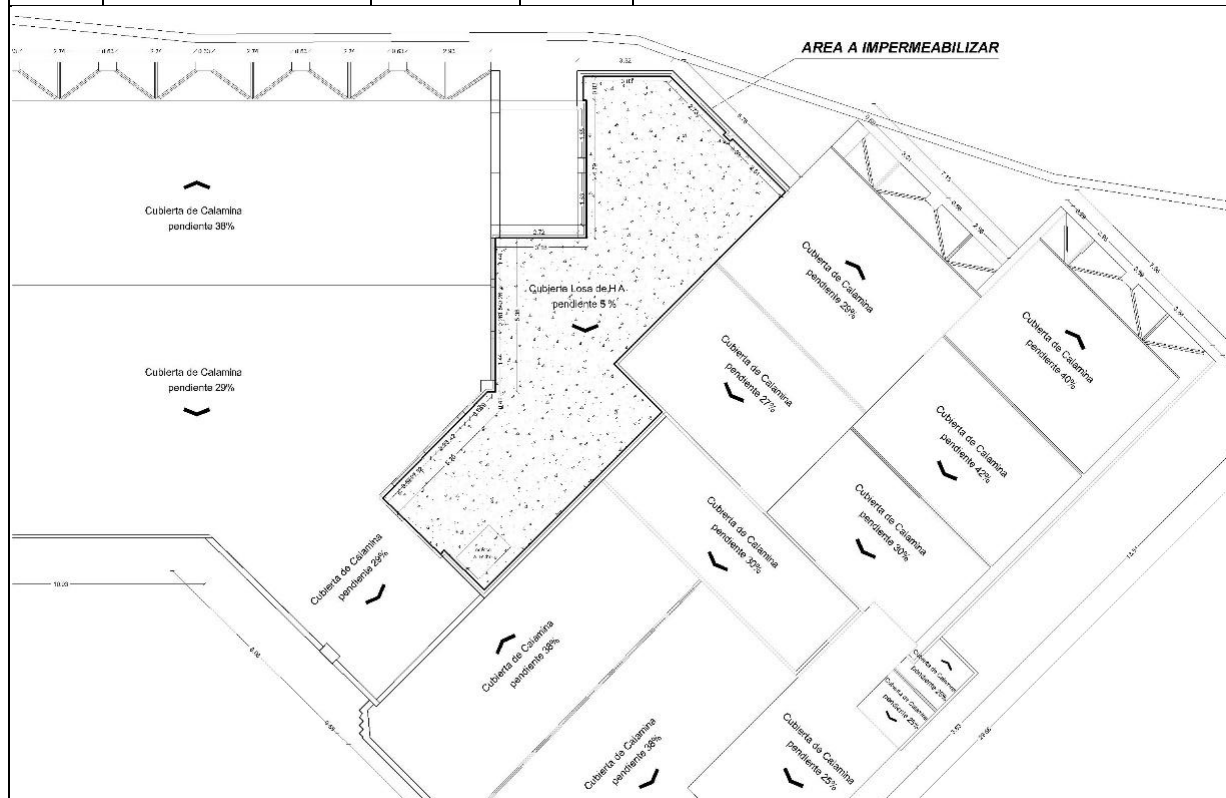
Figura Nro. 1 Vista del área a impermeabilizar de la Terraza Bloque D
